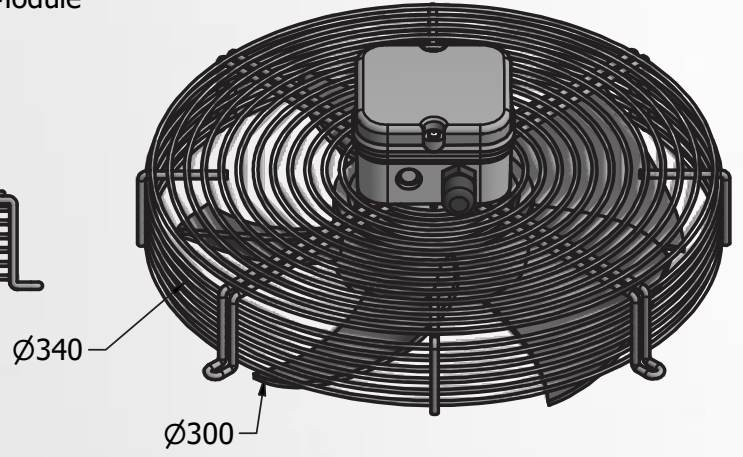
Fan Module
