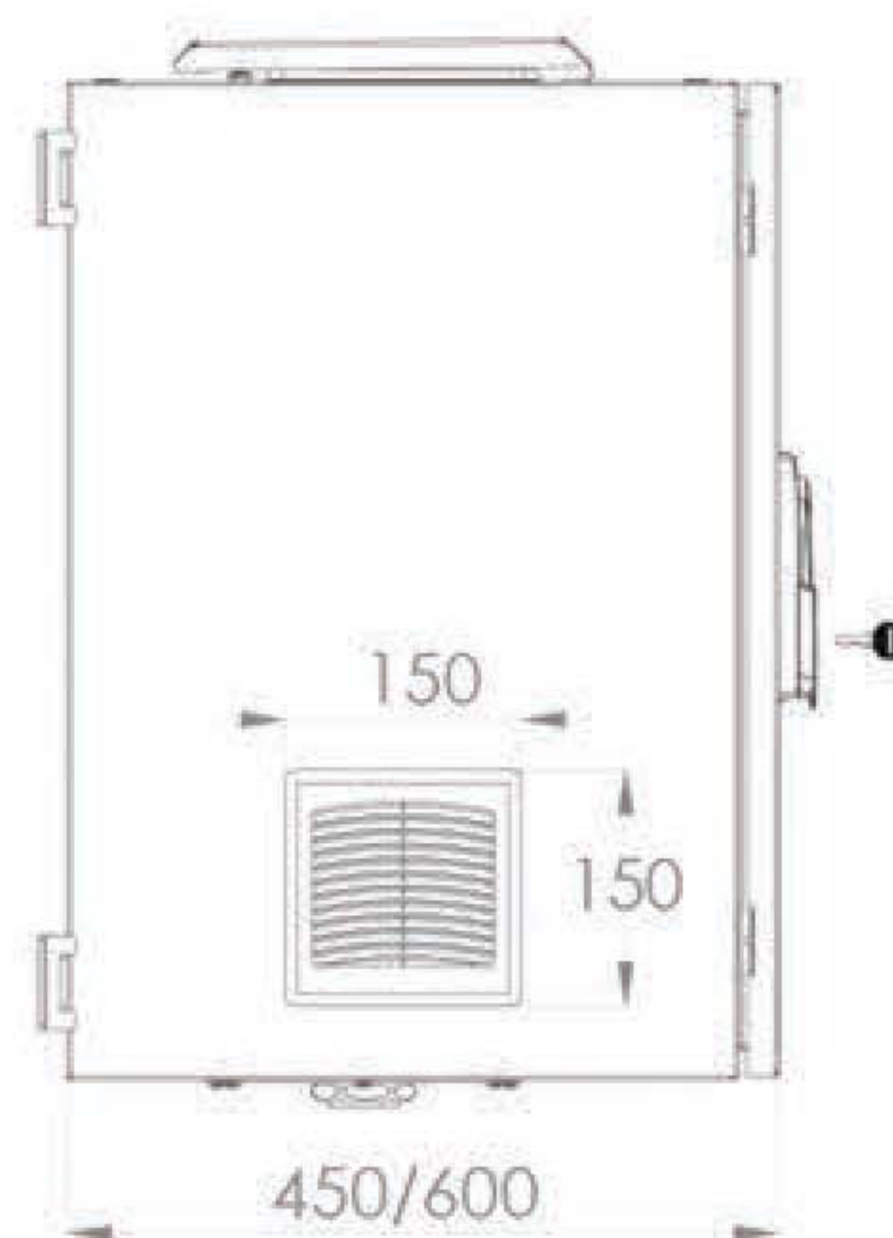
Vue de côté
