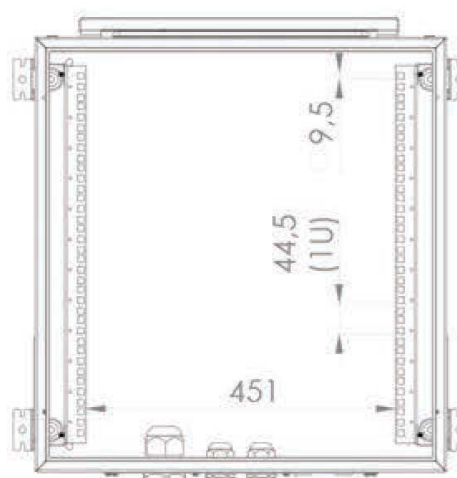
Vue de l'intérieur
