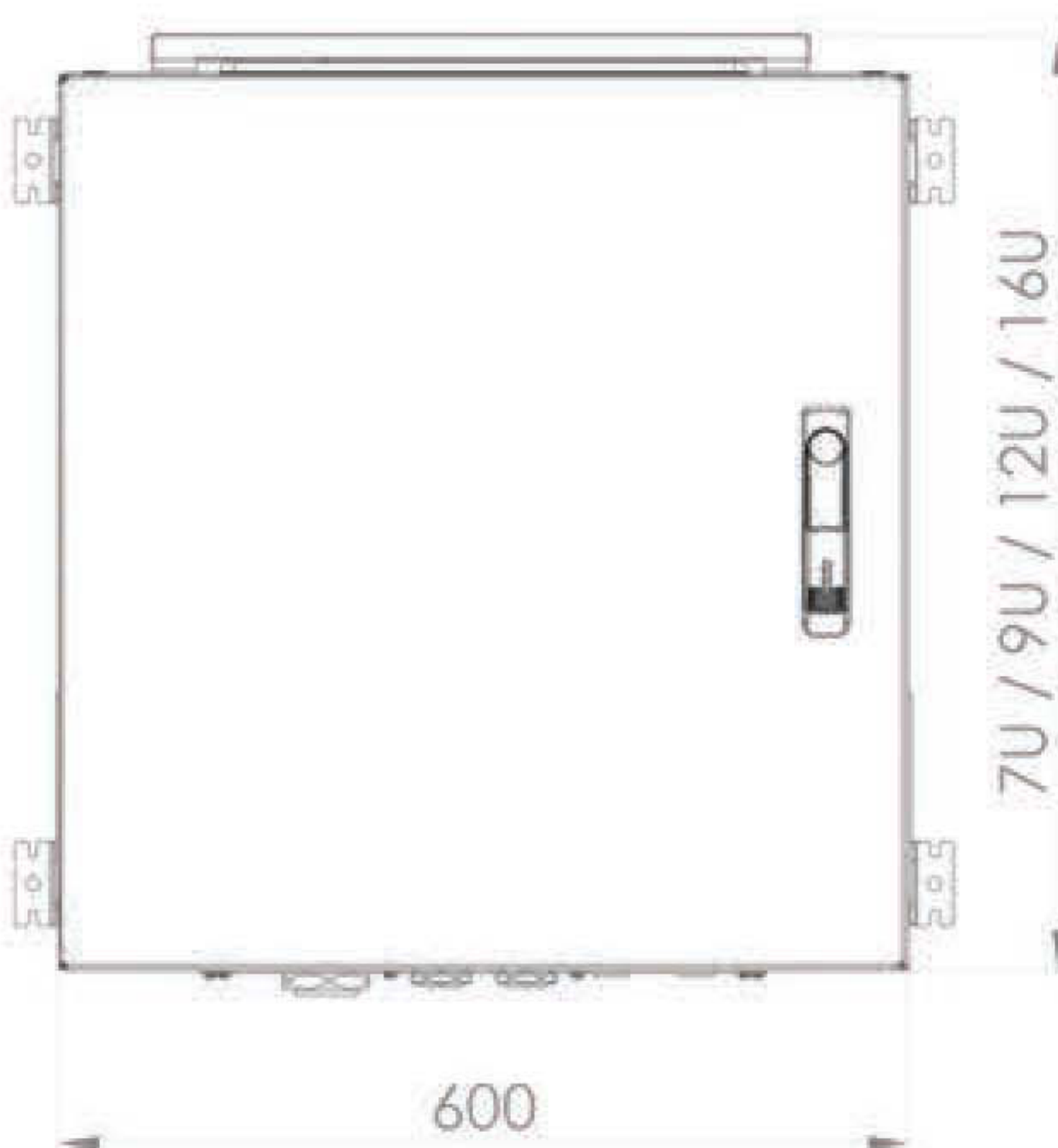
Vue de face
